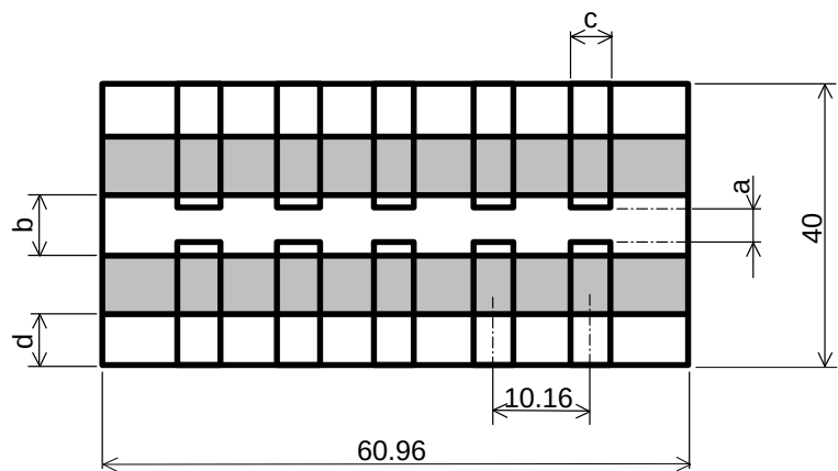
図-3 RZC50, 63 用 試験基板略図
