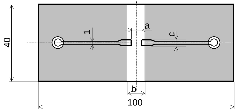
図-4 RZC50, 63 用 耐プリント板曲げ性 試験基板略図
