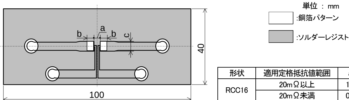
RCC16,20,32 用 耐プリント板曲げ性 試験基板略図
