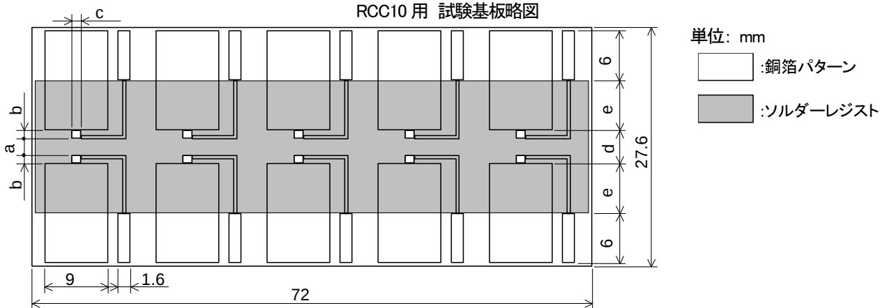
RCC10 用 試験基板略図
