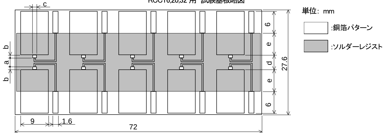
RCC16,20,32 用 試験基板略図
