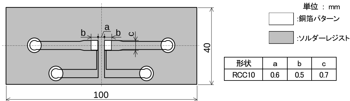
RCC10 用 耐プリント板曲げ性 試験基板略図
