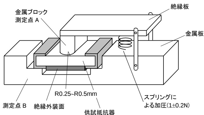
・RCC16, 20, 32 取付け図
