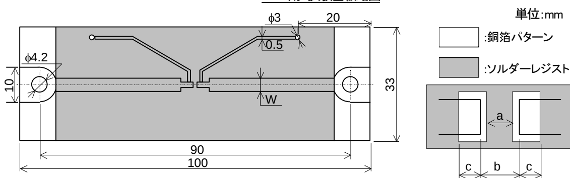
HFC 用 試験基板略図
