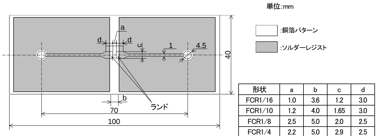
FCR 用 耐プリント板曲げ性 試験基板略図
