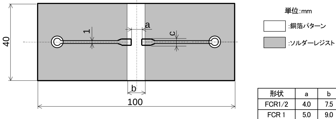
図-4 FCR1/2, 1 用 耐プリント板曲げ性 試験基板略図
