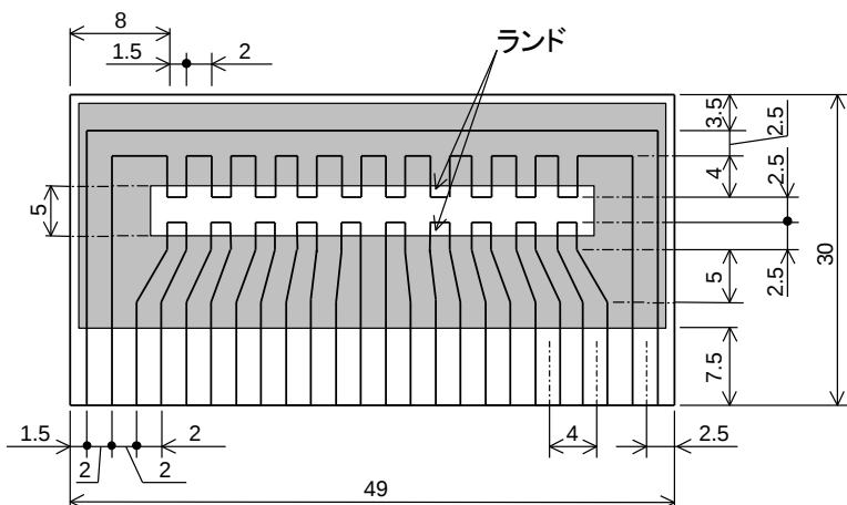
FCR1/8 用 試験基板略図
