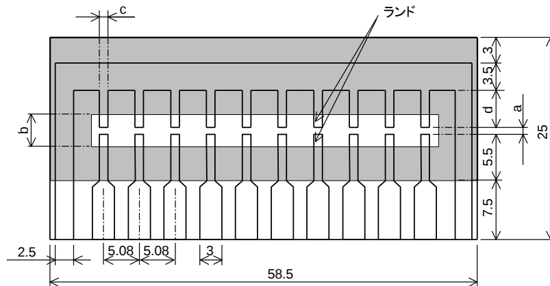
FCR1/8 用 試験基板略図
