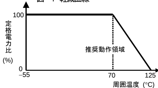
図-1 軽減曲線
