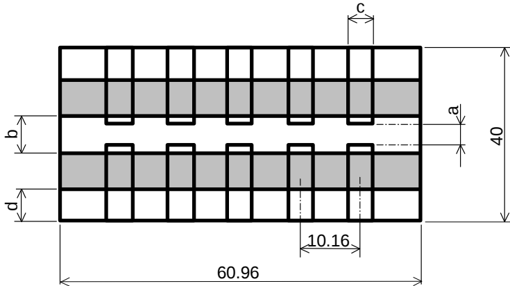
FCR1/2, 1 用 試験基板略図
