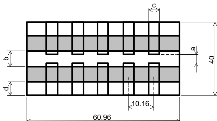
RPC50,63 用 試験基板略図
