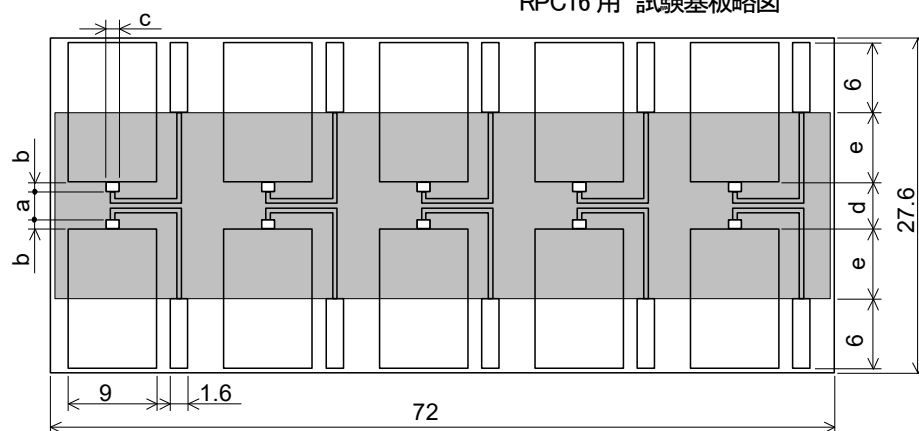
RPC16 用 試験基板略図
