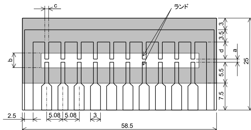
RPC20,32,35 用 試験基板略図
