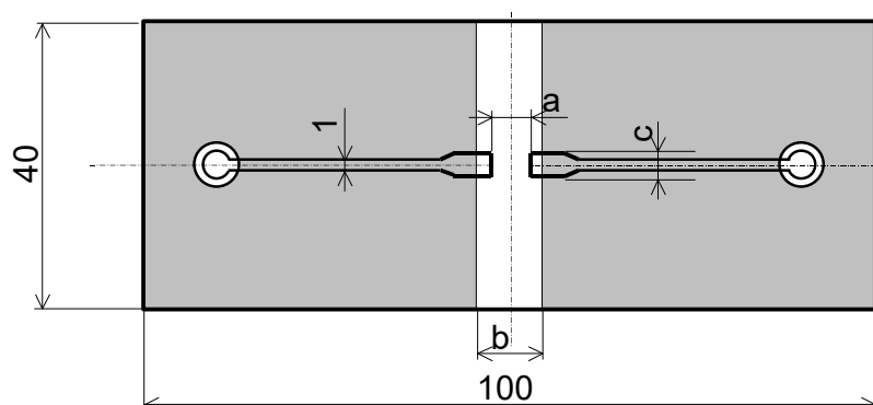
RPC16,20,32,35 用 耐プリント板曲げ性 試験基板略図
