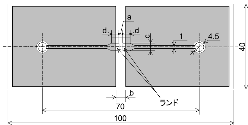
RPC16,20,32,35 用 耐プリント板曲げ性 試験基板略図
