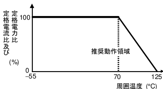
図-1 軽減曲線
