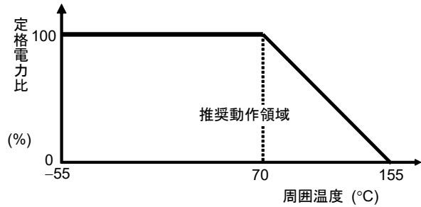
図-1 軽減曲線
