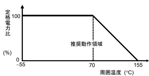
図－1 軽減曲線
